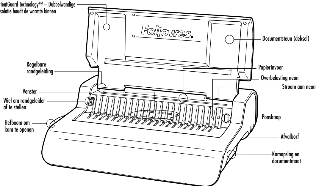
Afvalkorf
